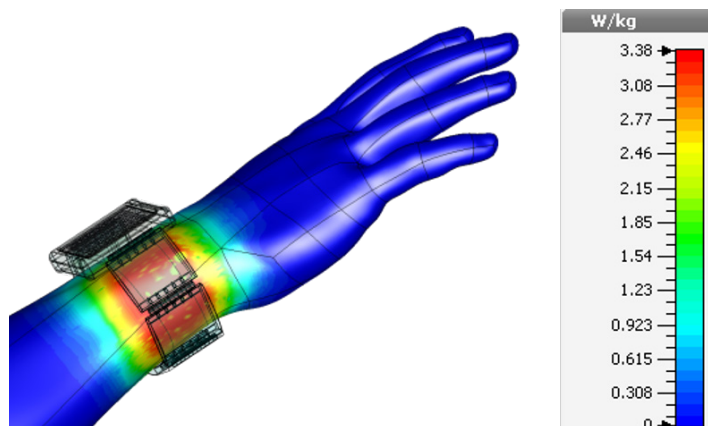
CST Berechnung EMAG: Abstrahlung Smart-Watch
