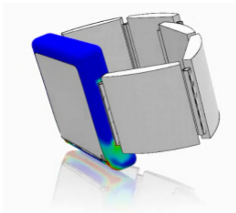
Abaqus Berechnung Strukturmechanik: Beispiel Drop-Test Smart-Watch
