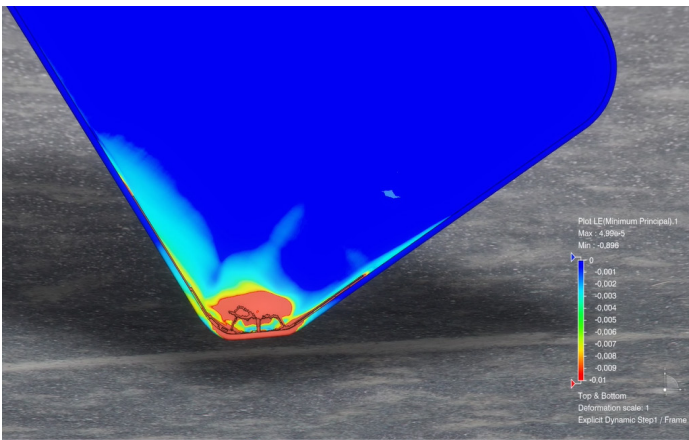
Abaqus Berechnung Strukturmechanik: Drop-Test Handy
