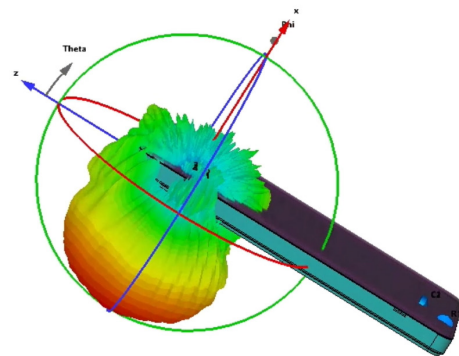
CST Berechnung EMAG: Abstrahlung Handy
